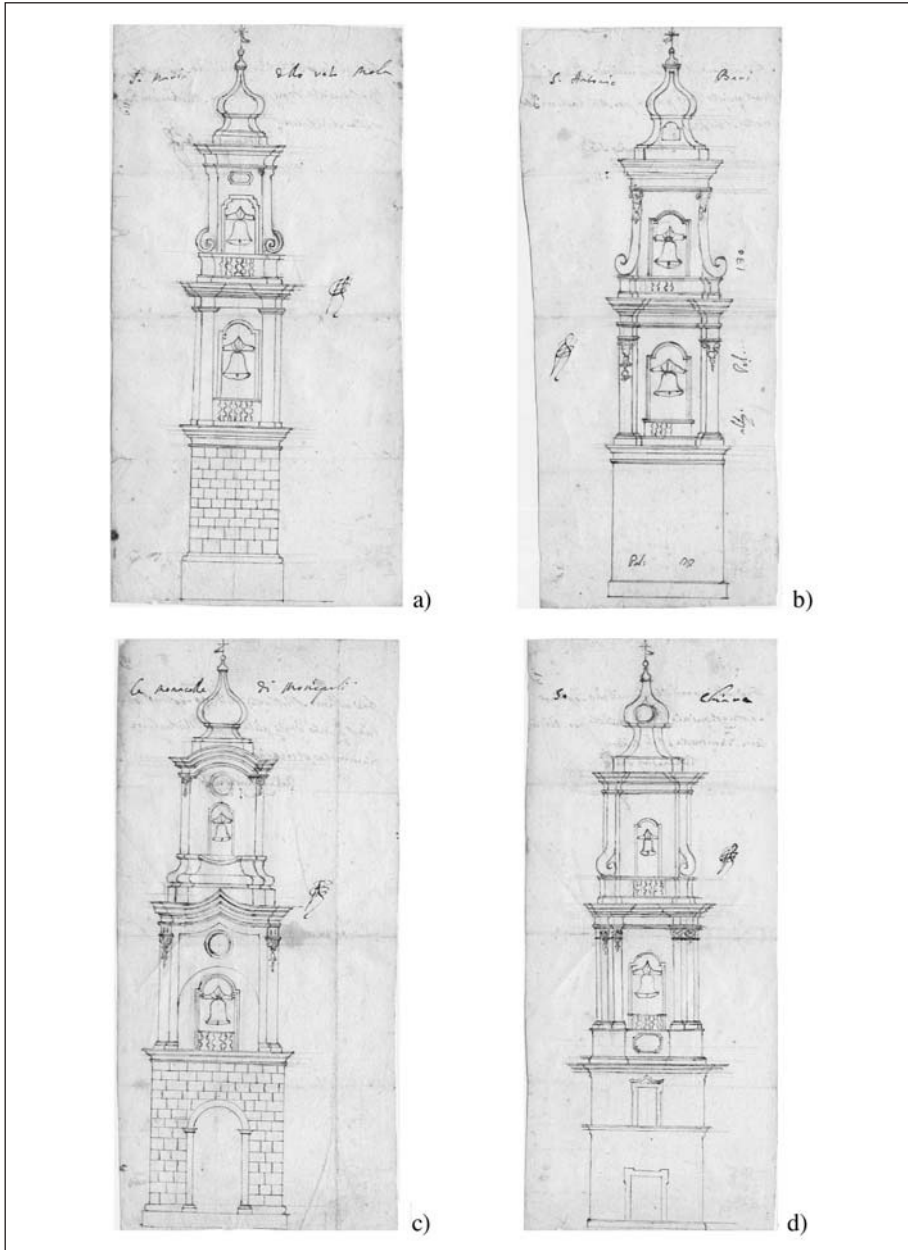
Fig. 1. Vito Ieva (attribuzione). Rilievi settecenteschi di campanili in Terra di Bari, 1760. (Asfg, Dogana II , F. 494, f. 10511):
