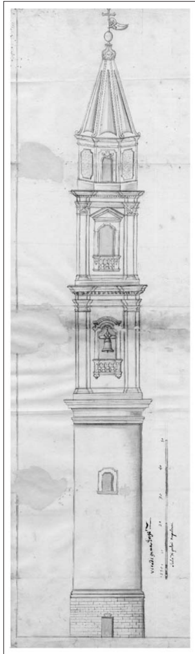
Fig. 2. Vito Ieva. Progetto per il campanile di S. Francesco in Andria, senza data, scala grafica in palmi napoletani, cm 38 x 134, b.n., restaurato (Asfg, Dogana II , F. 494, f. 10511, cc. 141-144). Concessione del Ministero per i Beni e le Attività Culturali – Archivio di Stato di Foggia.
