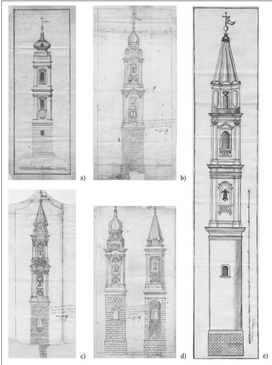
Fig. 3. Progetti settecenteschi di campanili barocchi (Asfg, Dogana II , F. 494, f. 10511): a) ignoto, senza data, scala grafica, cm 17 x 38, b.n., restaurato (c. 139); b) ignoto, senza data, scala grafica, cm 29 x 54, b.n., restaurato (c. 52); c) ignoto, datato 1765, scala grafica, cm 35 x 72, b.n., restaurato (c. 53); d) ignoto, senza data, scala grafica, cm 24 x 37, b.n., restaurato (c. 56); e) Francesco Matrella, senza data, scala grafica, cm 15 x 68, b.n., restaurato (c. 92). Concessione del Ministero per i Beni e le Attività Culturali – Archivio di Stato di Foggia.
